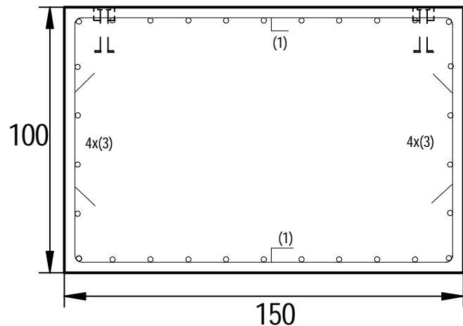
Langsdoorsnede
