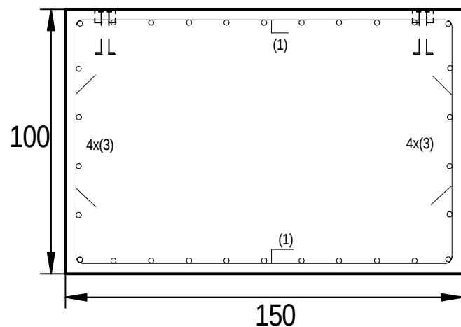
Langsdoorsnede
