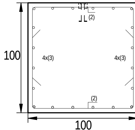
Dwarsdoorsnede
